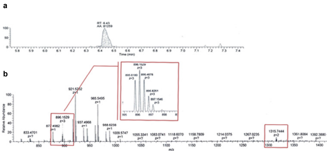
Figura 1. Cromatogramma estratto di ioni bicarica e tricarica ( Extracted Ion Chromatogram , XIC) dell'ovatossina-a in un campione di aerosol raccolto nell'agosto 2010 lungo le coste toscane (a) e lo spettro di massa ad alta risoluzione (HRMS) associato (b)
